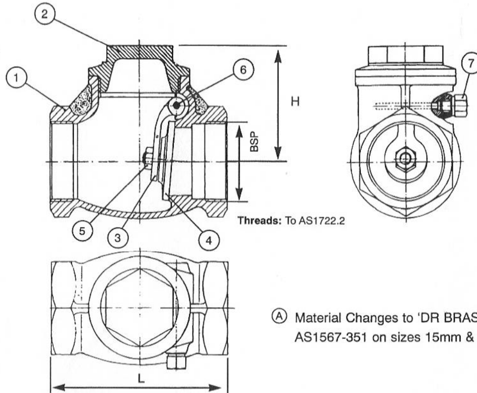
Dimensions
